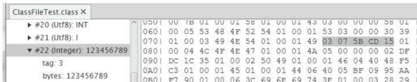
图3-9 用classpy观察CONSTANT_Integer_info常量
