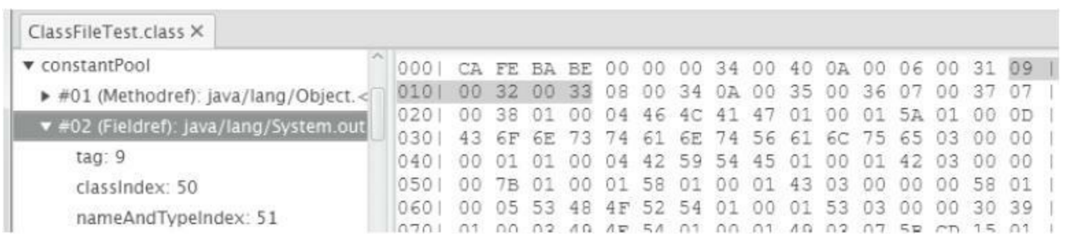
图3-18 用classpy观察CONSTANT_Fieldref_info常量
