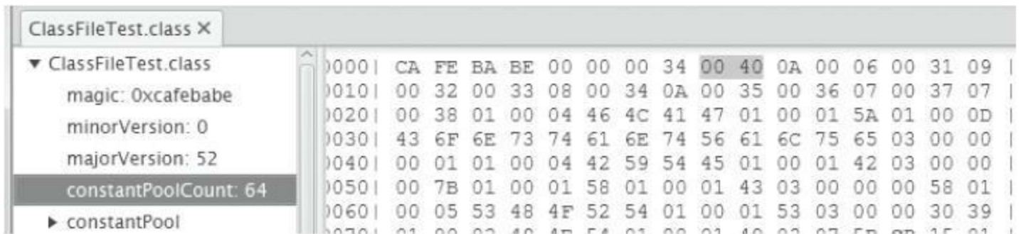
图3-8 用classpy观察常量池大小
