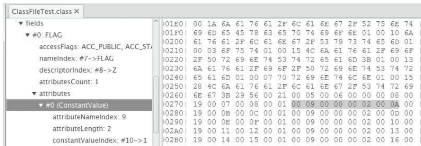
图3-23 用classpy观察ConstantValue属性
