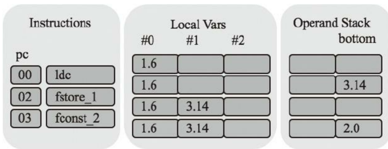
图4-6 circumference()方法执行示意图(4)
