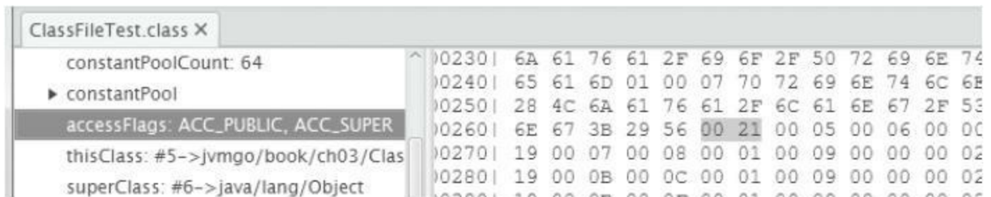
图3-3 用classpy观察类访问标志
