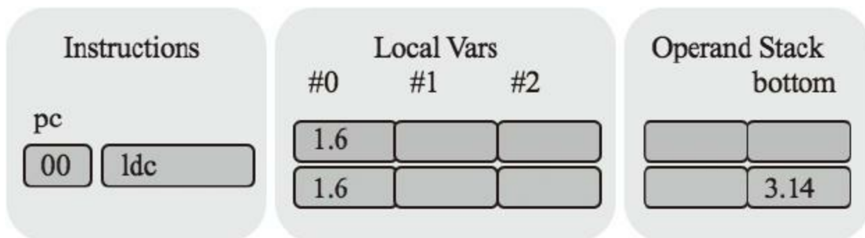
图4-4 circumference()方法执行示意图(2)
