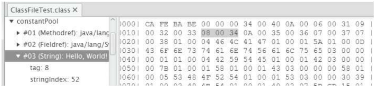
图3-14 用classpy观察CONSTANT_String_info常量
