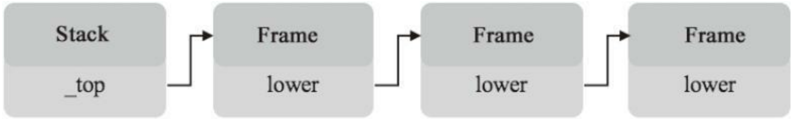
图4-2 使用链表实现Java虚拟机栈
