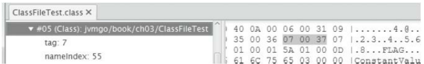
图3-16 用classpy观察CONSTANT_Class_info常量
