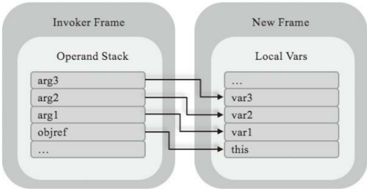
图7-2 实例方法参数传递示意图
