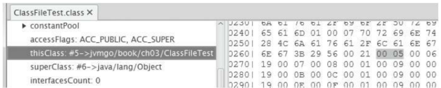
图3-4 用classpy观察类和超类索引
