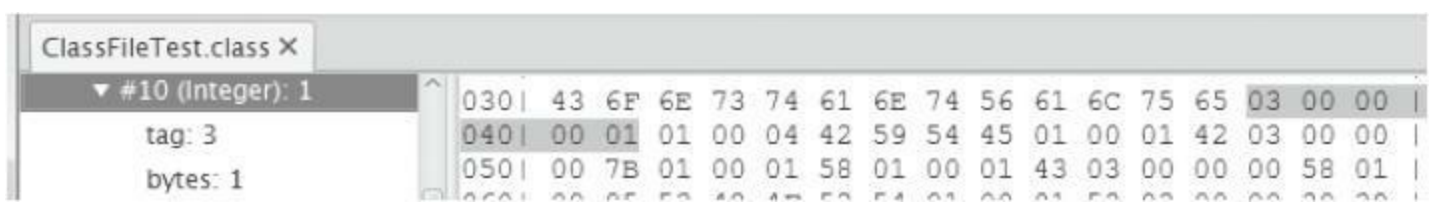
图3-24 用classpy观察ConstantValue属性(2)
