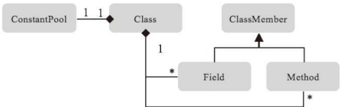
图6-1 Class结构体关系图
