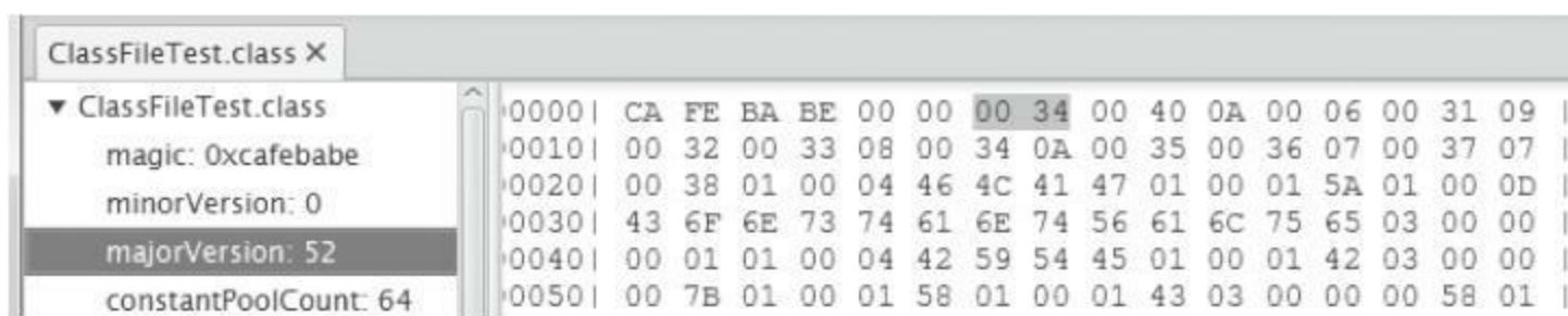
图3-2 用classpy观察版本号
