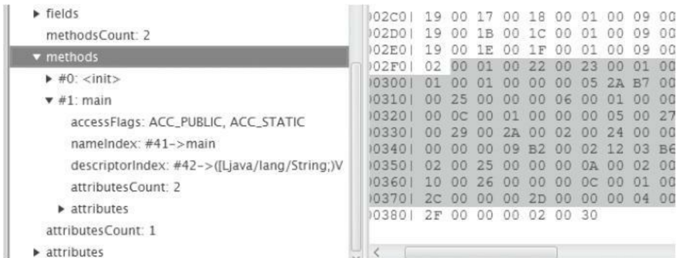
图3-7 用classpy观察方法表
