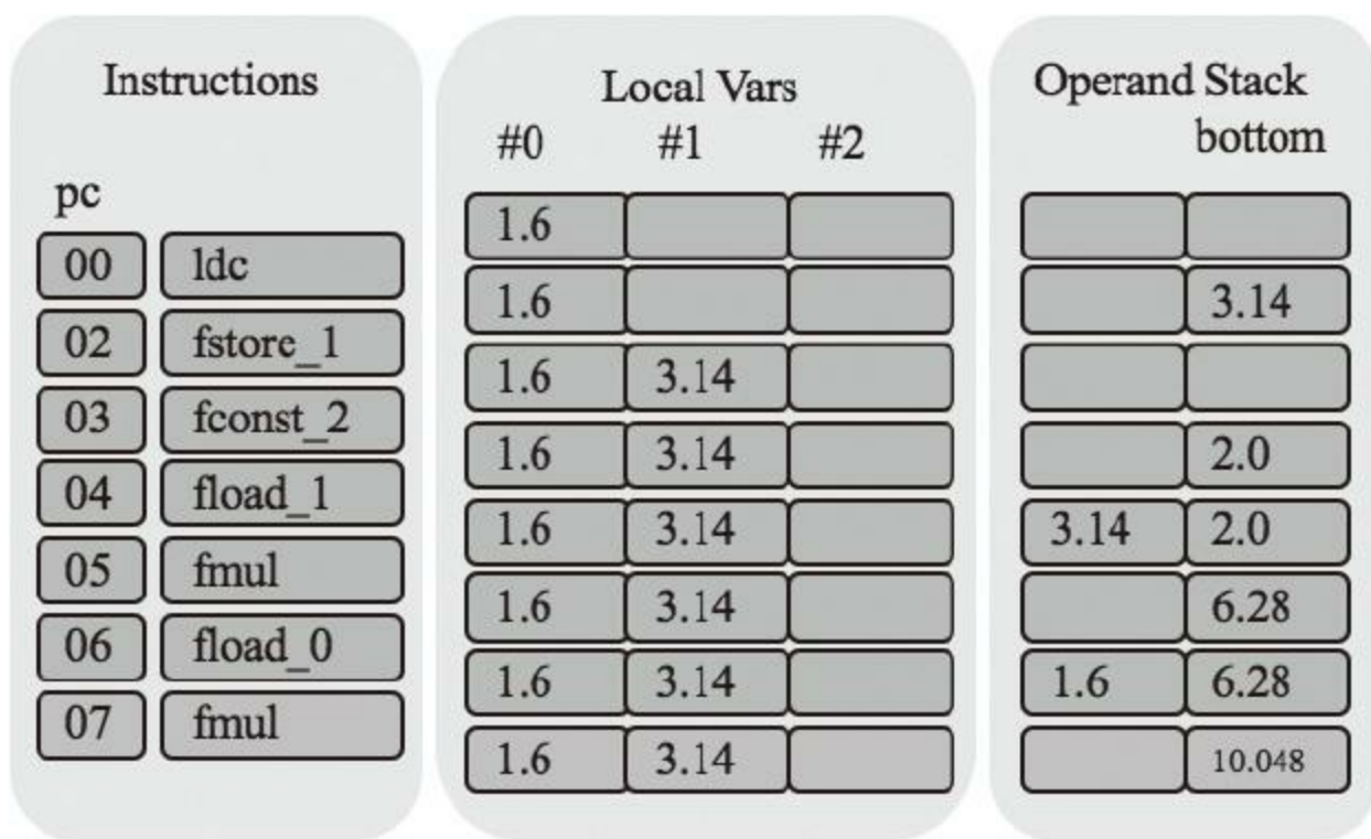
图4-10 circumference()方法执行示意图(8)
