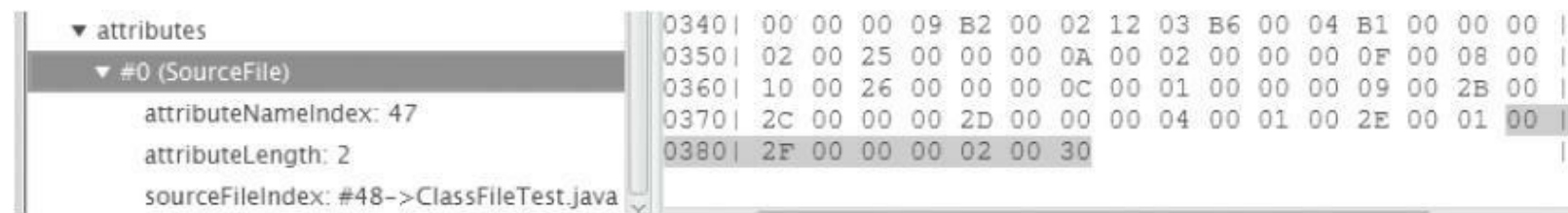
图3-21 用classpy观察SourceFile属性
