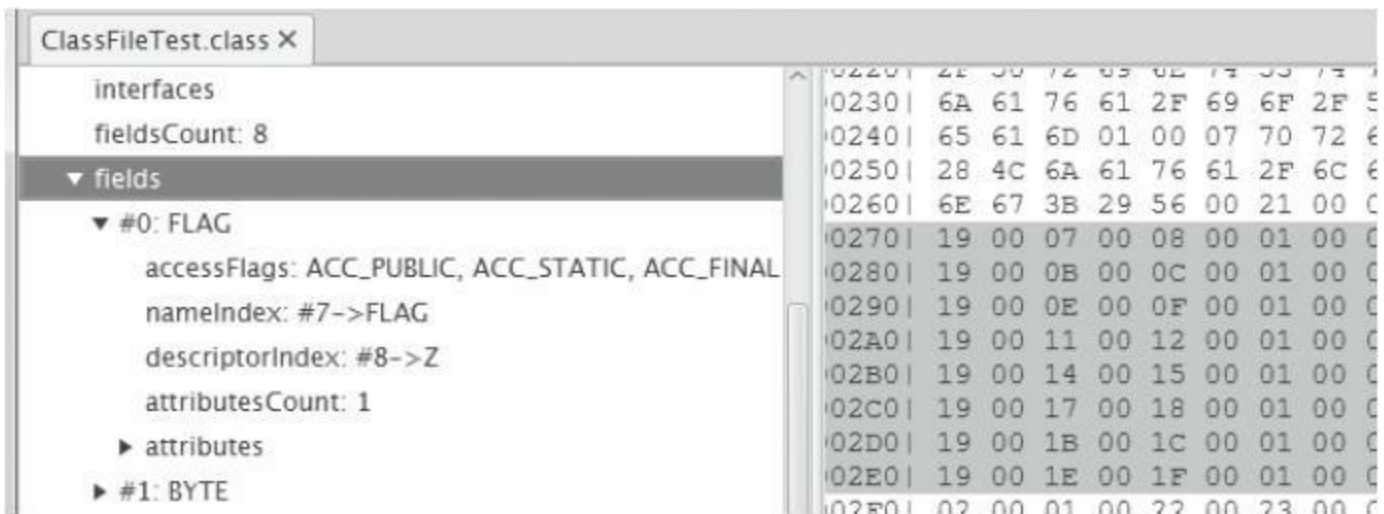
图3-6 用classpy观察字段表
