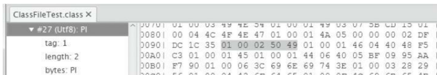
图3-13 用classpy观察CONSTANT_Utf8_info常量
