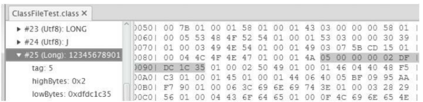
图3-11 用classpy观察CONSTANT_Long_info常量
