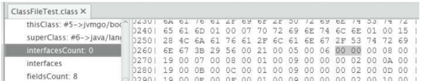
图3-5 用classpy观察接口索引表
