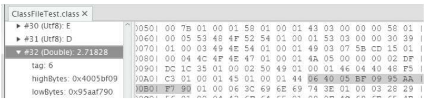
图3-12 用classpy观察CONSTANT_Double_info常量
