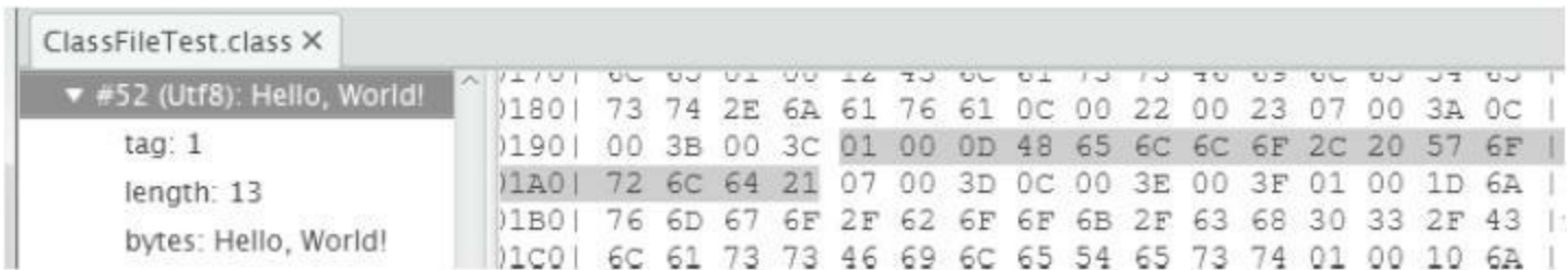
图3-15 用classpy观察CONSTANT_String_info常量(2)
