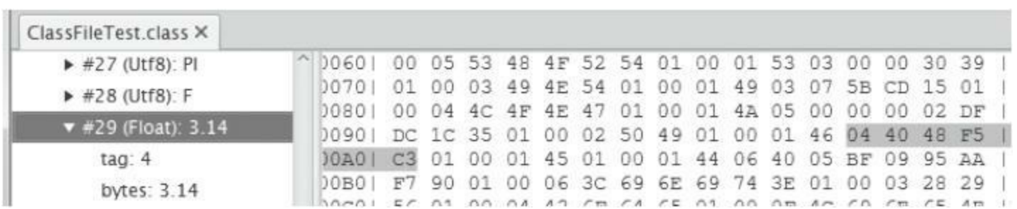
图3-10 用classpy观察CONSTANT_Float_info常量
